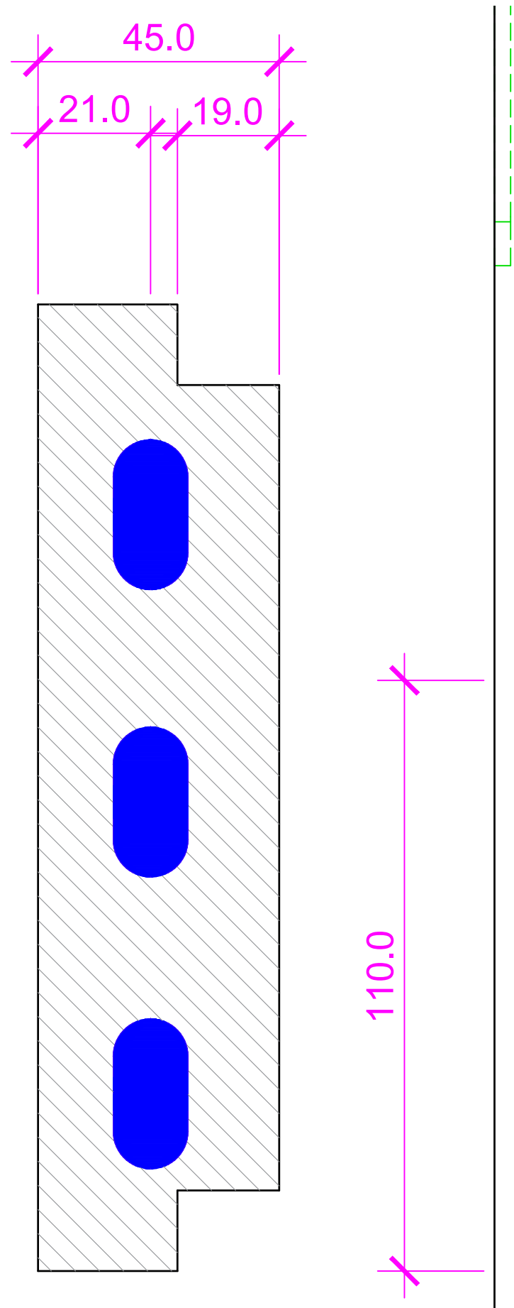
Türrahmen Detail 1:1 3.2.21
