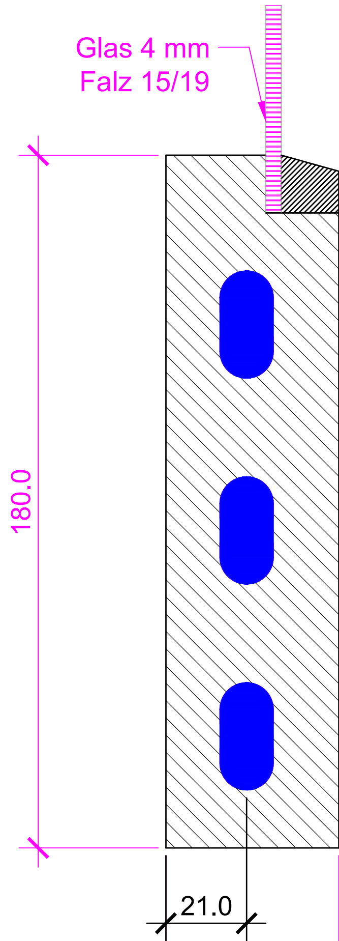
Türrahmen Detail 1:1 3.2.21
