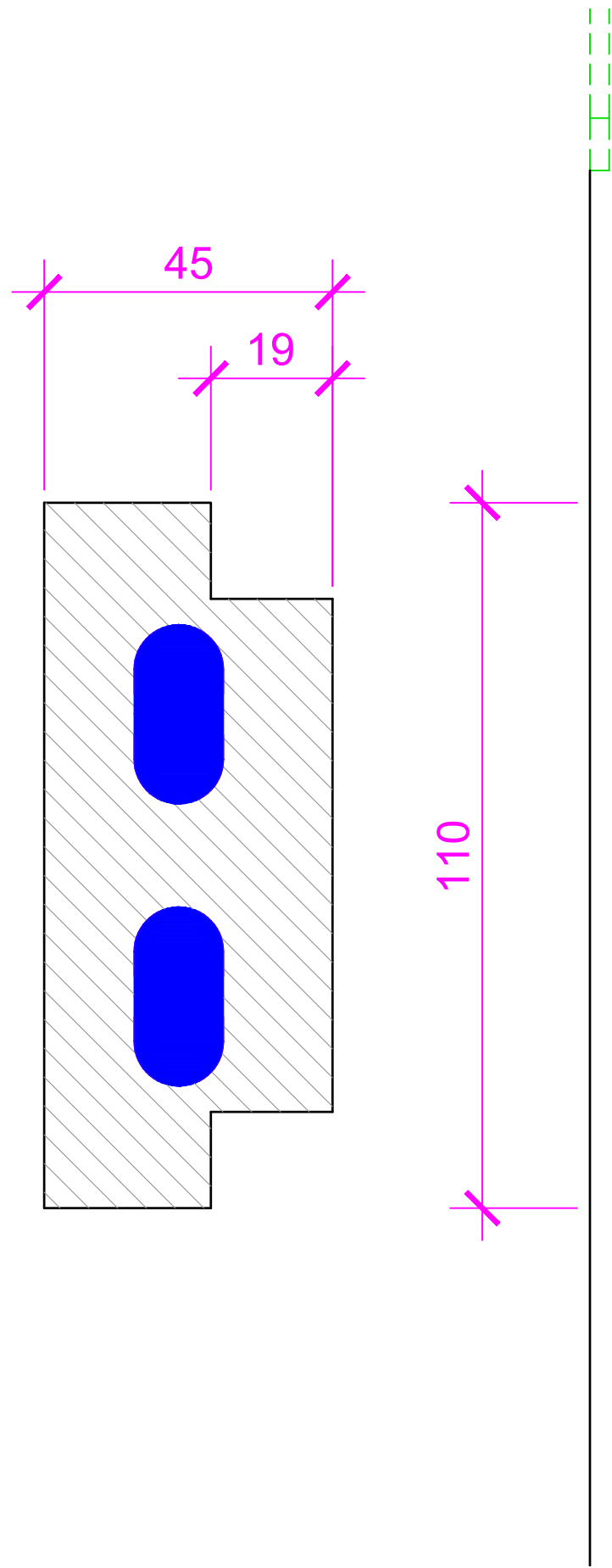
Türrahmen Detail 1:1 3.2.21
