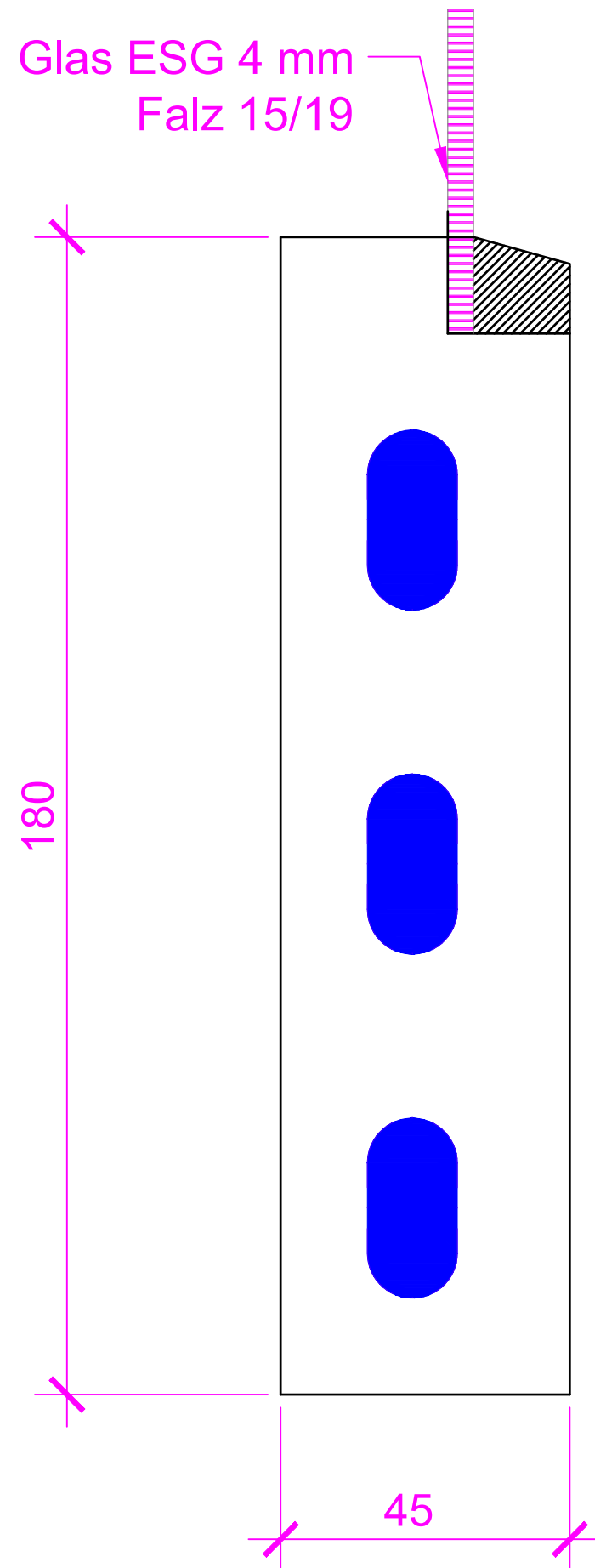
Türrahmen Detail 1:1 3.2.21
